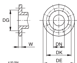
Flansche EN 1092-2
